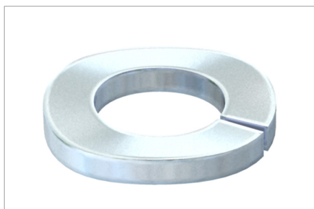
Inel spiralat conform DIN 128 forma A.
